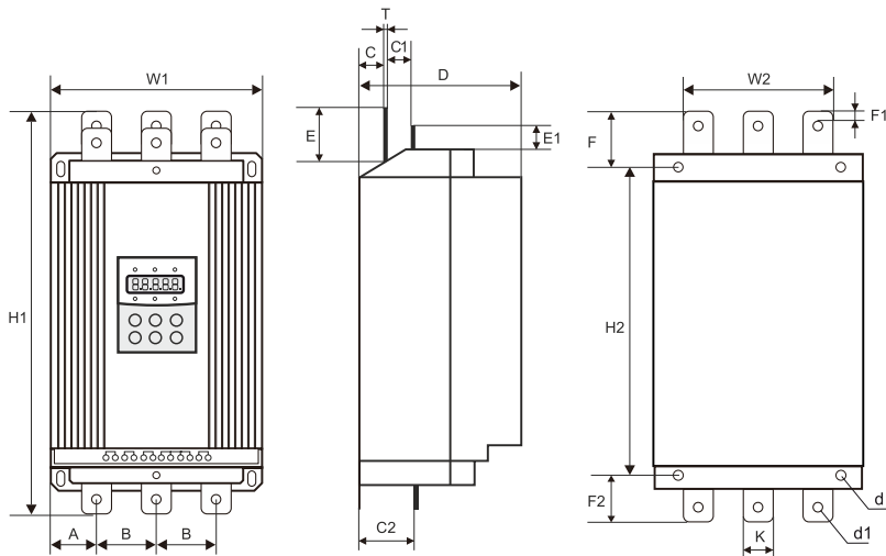
Типоразмеры, мм
